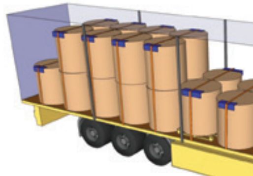
Figur 34: Panelblokering med lastpalle
