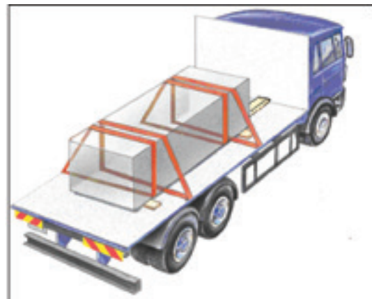
Figur 38: Halv kædesurring
