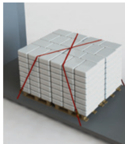
Figur 72: Fire paller med krydssurring
